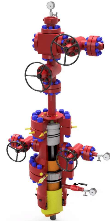
Cabezal Estándar 10 KSI/15 KSI API 6A PSL3 PR2
